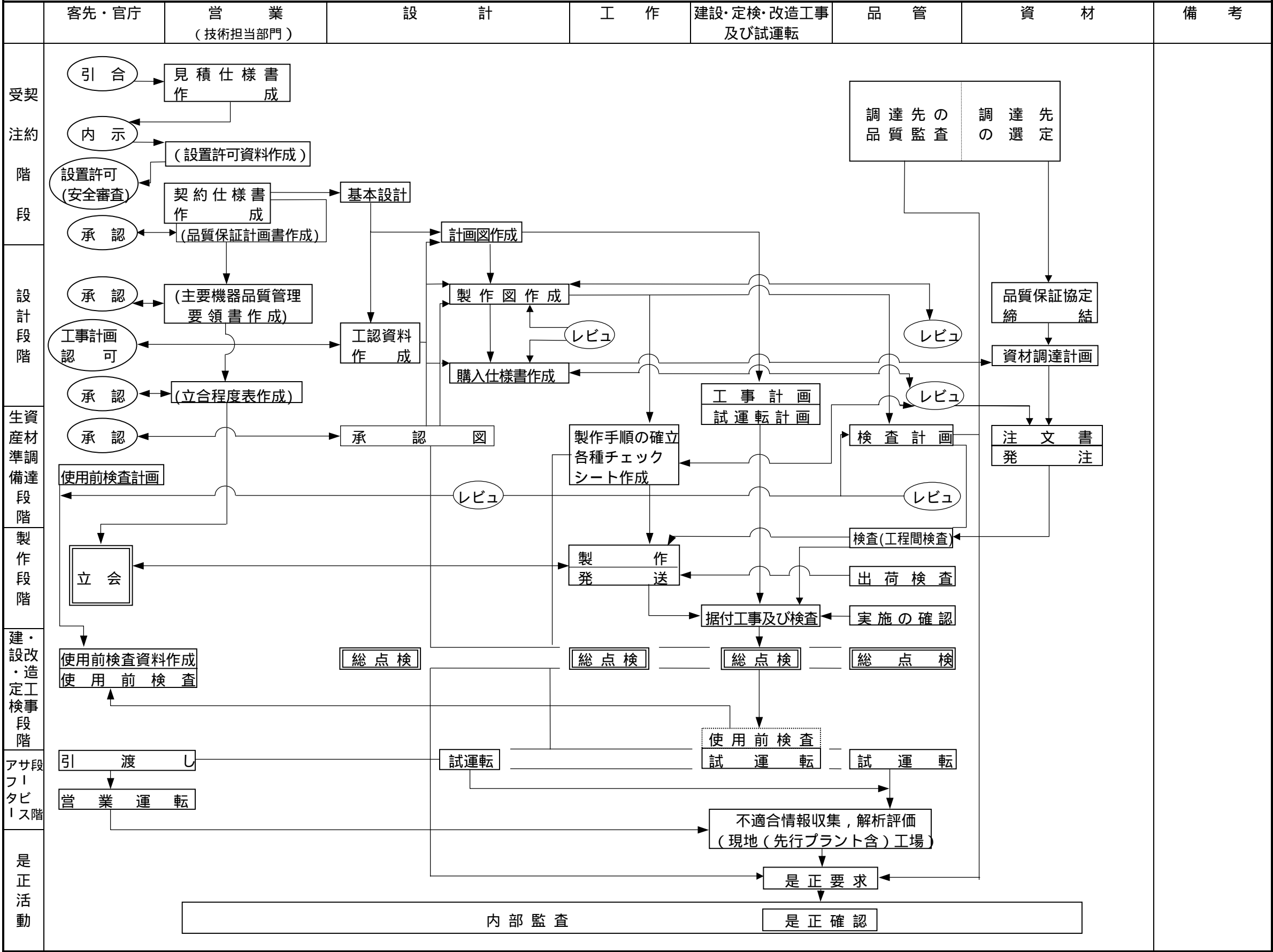
参考図5 電力・産業システム事業所 品質保証機能体系図
