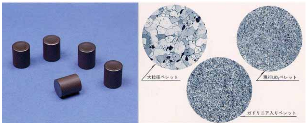
UO 2 ペレット外観
