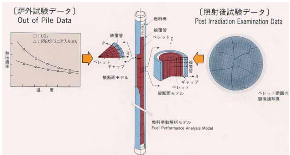
参考図 6 燃料試験データと解析モデルの例
