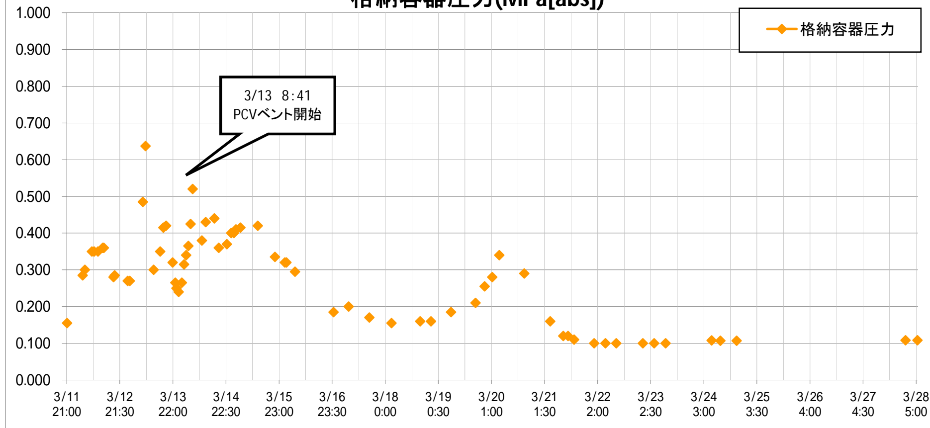
格納容器圧力 (MPa[abs])
