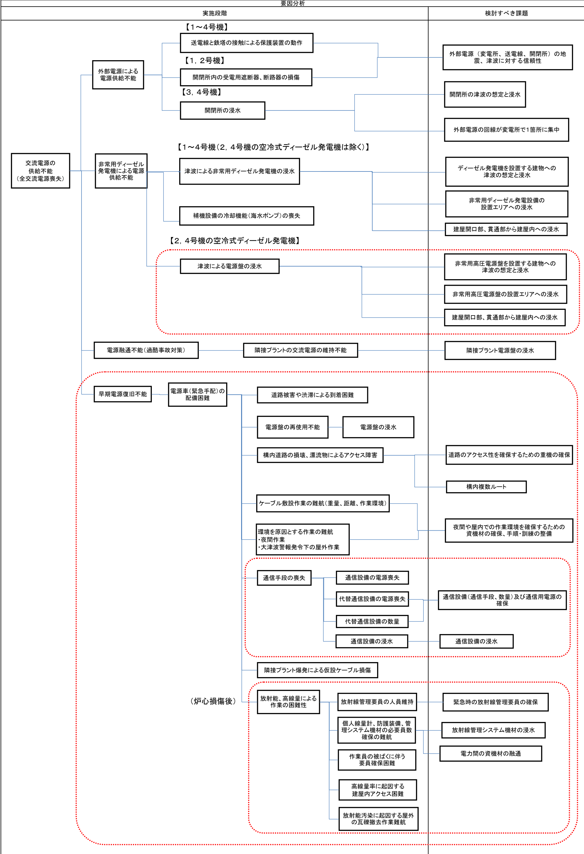
図 2.2.1 交流電源供給不能 原因分析
